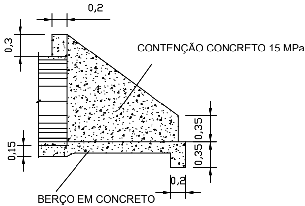
VISTA LATERAL BOCA DE ALAS
