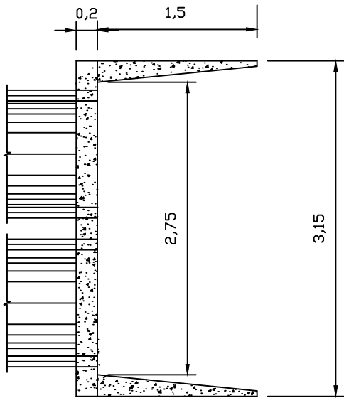
PLANTA BAIXA BOCA DE ALAS
