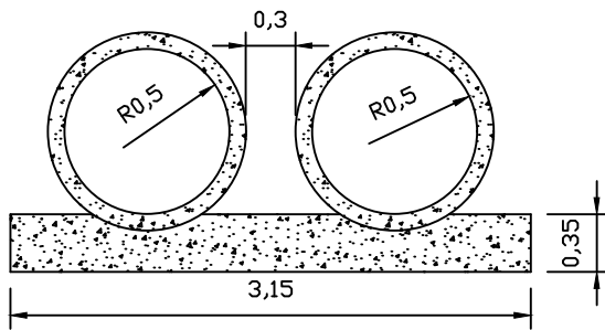
CORTE BUEIRO
